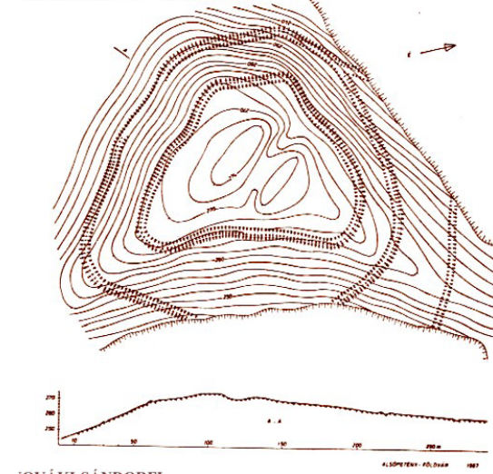
Forrás: Gádor Judit
